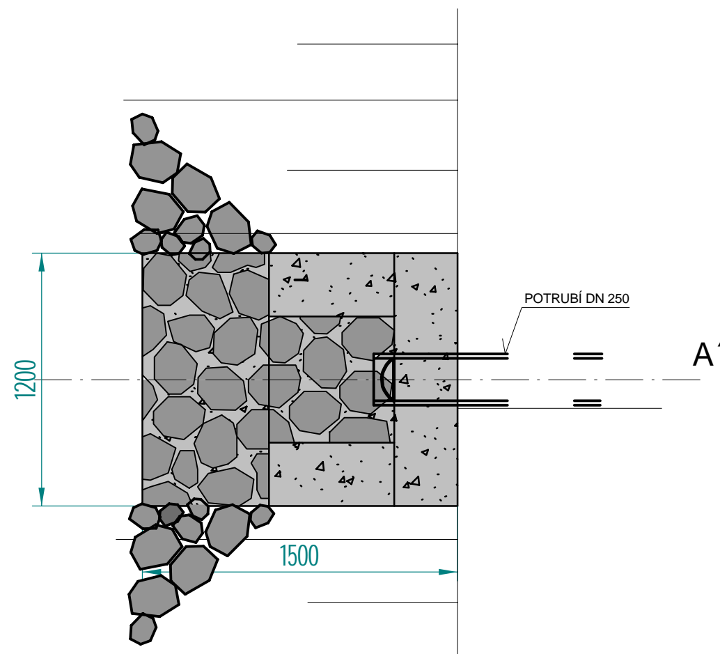
PŮDORYS
